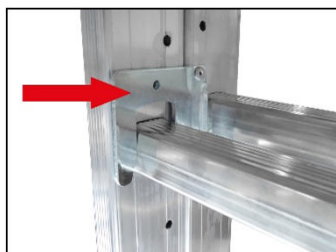
Bild 2 (fehlerfrei)
