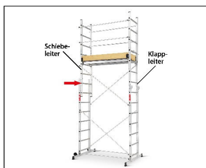
Bild 1 (fehlerhaftes Leiterteil)
